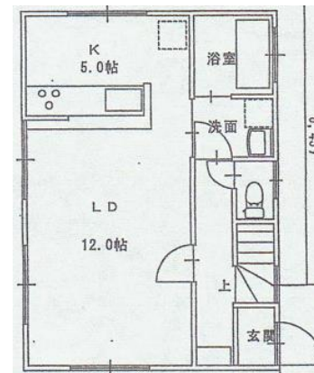
1階平面図
