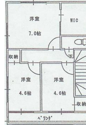
2階平面図
